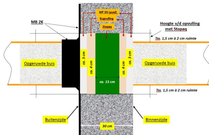
Fig. 3 – detail waterdichting buisdoorvoer - afdichting rond de buis
