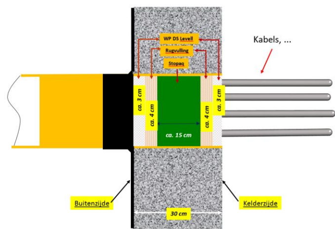
Fig. 4 – detail waterdichting buisdoorvoer - afdichting in de buis
