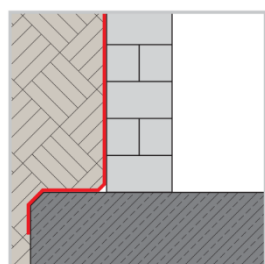
afdichting ondergrondse structuur
