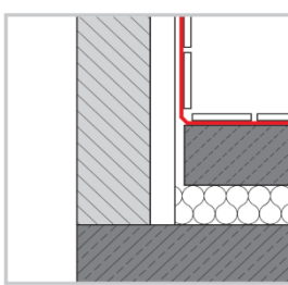
afdichting onder tegels in natte ruimten en voor terrassen en balkons
