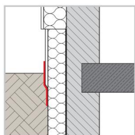
Fig. 1 – Mogelijke toepassingen van het waterdichtingssysteem
