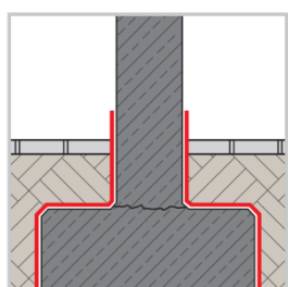
afdichting van funderingen
